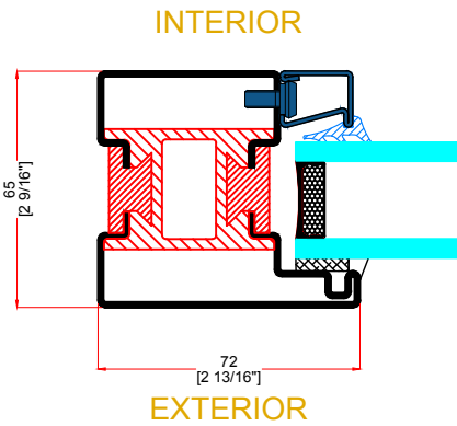
1 OPTIONAL FIXED JAMB
