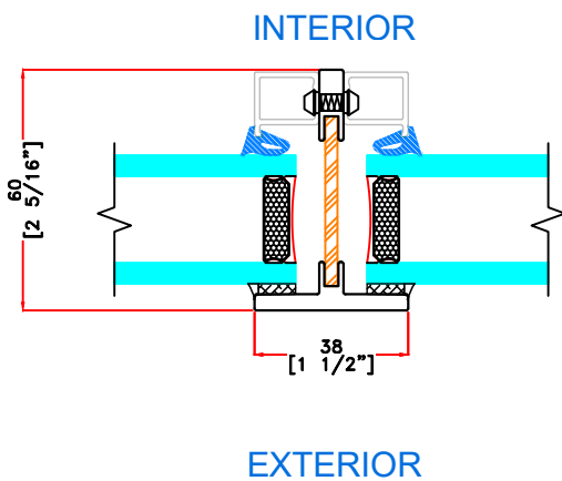
P OPTIONAL VERTICAL MUNTIN
