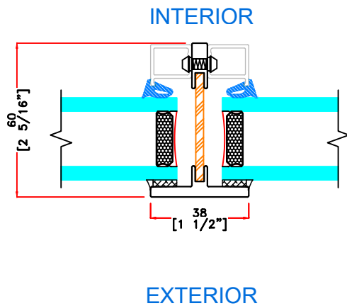
P OPTIONAL VERTICAL MUNTIN
